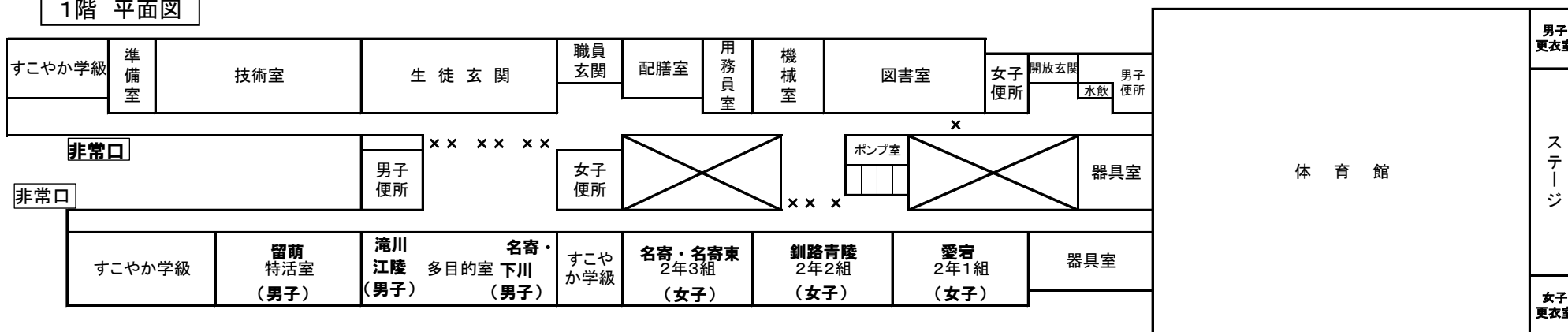
1階 平面図
