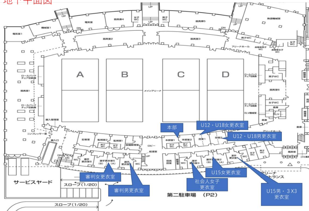
地下平面図
